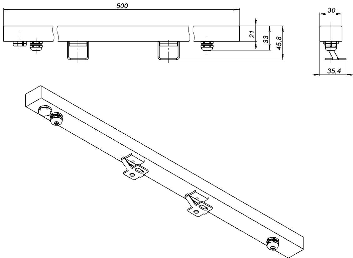
Рисунок 1. Общий вид светильника RAD-L-SL
